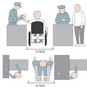
检票口和结算口图示
