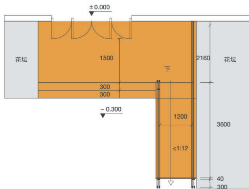
同时设置台阶和轮椅坡道的出入口图示
