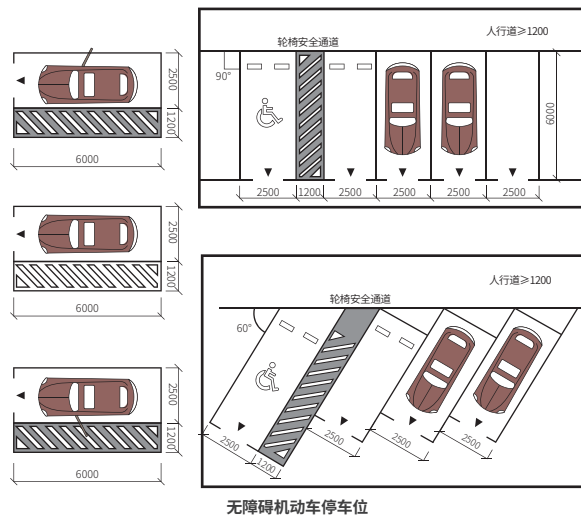
无障碍机动车停车位
