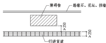
① 盲道遇障碍物平面布置
