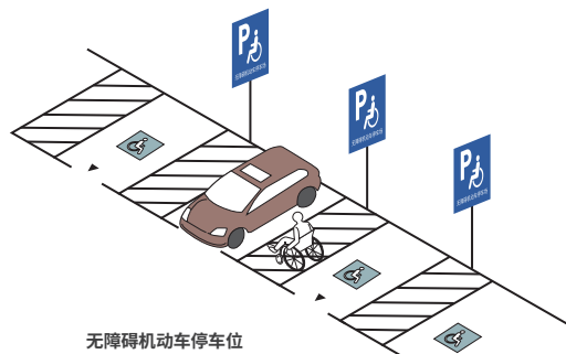
无障碍机动车停车位
