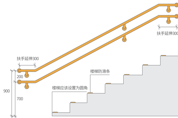
楼梯示意图
