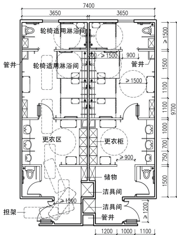
无障碍公共浴室平面示例
