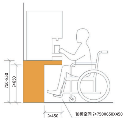
低位服务设施图示
