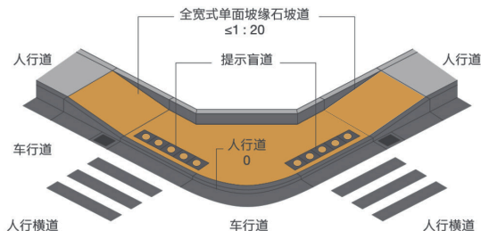
全宽式单面坡缘石坡道图示
