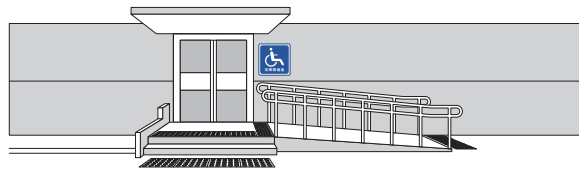
直线型轮椅坡道图示
