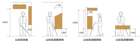
盲杖探各处障碍物图示
