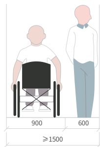
无障碍通道宽度图示
