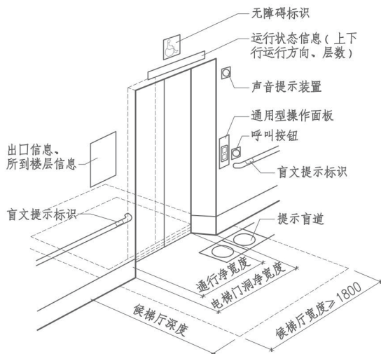
无障碍候梯厅图示
