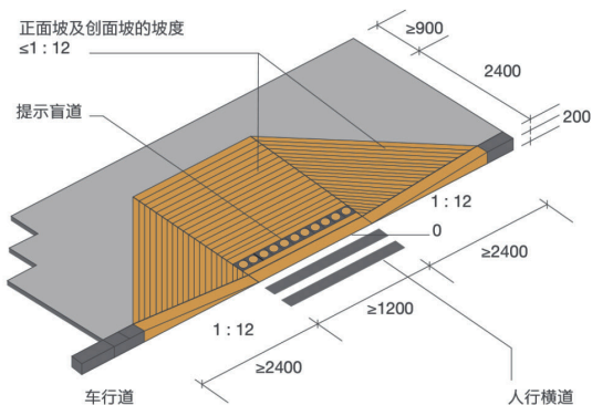
三面坡缘石坡道图示
