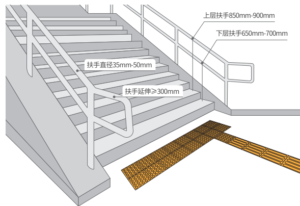
台阶示意图
