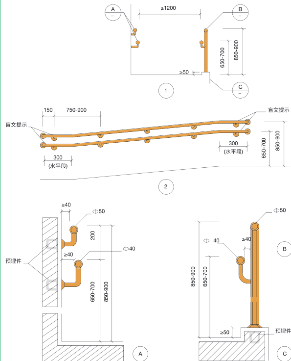
坡道扶手图示
