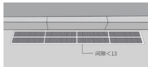
雨水箅子示意图
