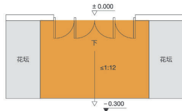
平坡出入口图示
