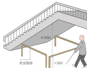
保护区示意图
